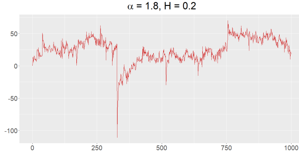
Slika 2. Trajektorija dobro balansiranog LFSG za \alpha = 1.8 i H = 0.2
