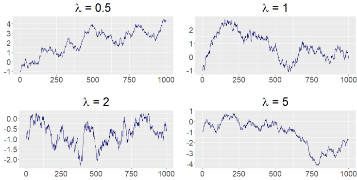
Slika 4. Trajektorije OU procesa za različite \lambda
