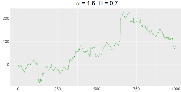
Slika 1. Trajektorija dobro balansiranog LFSG za \alpha = 1.6 i H = 0.7
