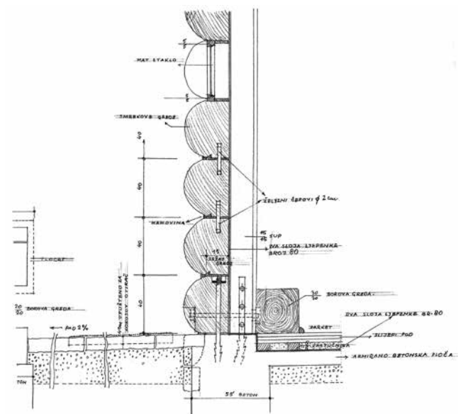
14a–b Vojta Braniš, Đuka Kavurić, Edo Kovačević, Đorđe Krekić i Ernest Tomašević, Nacrti (tlocrt, presjeci, opločenje poda, strop i detalj vanjskog zida). Bosanska kuća na Svjetskoj izložbi u Parizu 1937., 1937. (privatno vlasništvo)
